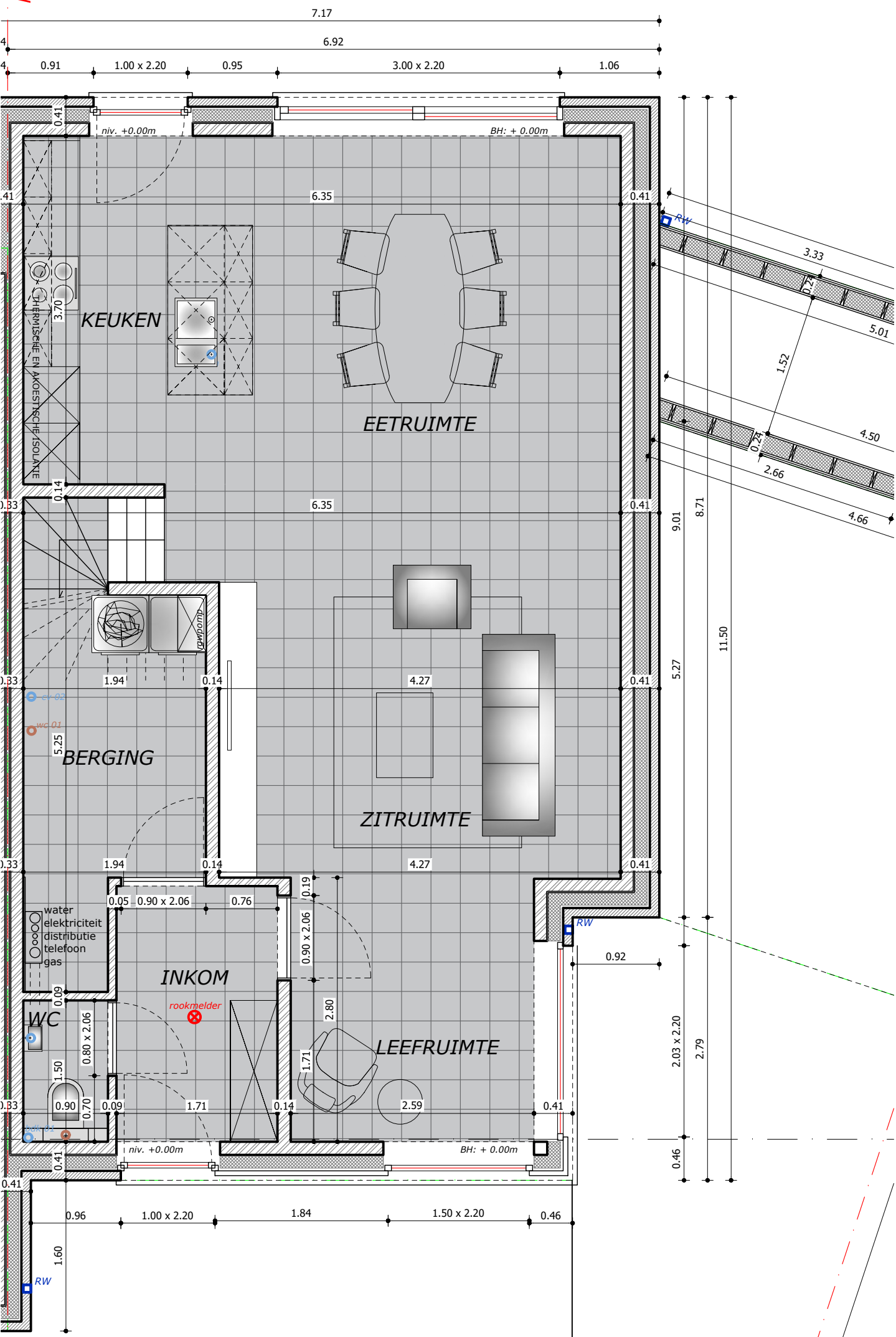
Gelijkvloers
