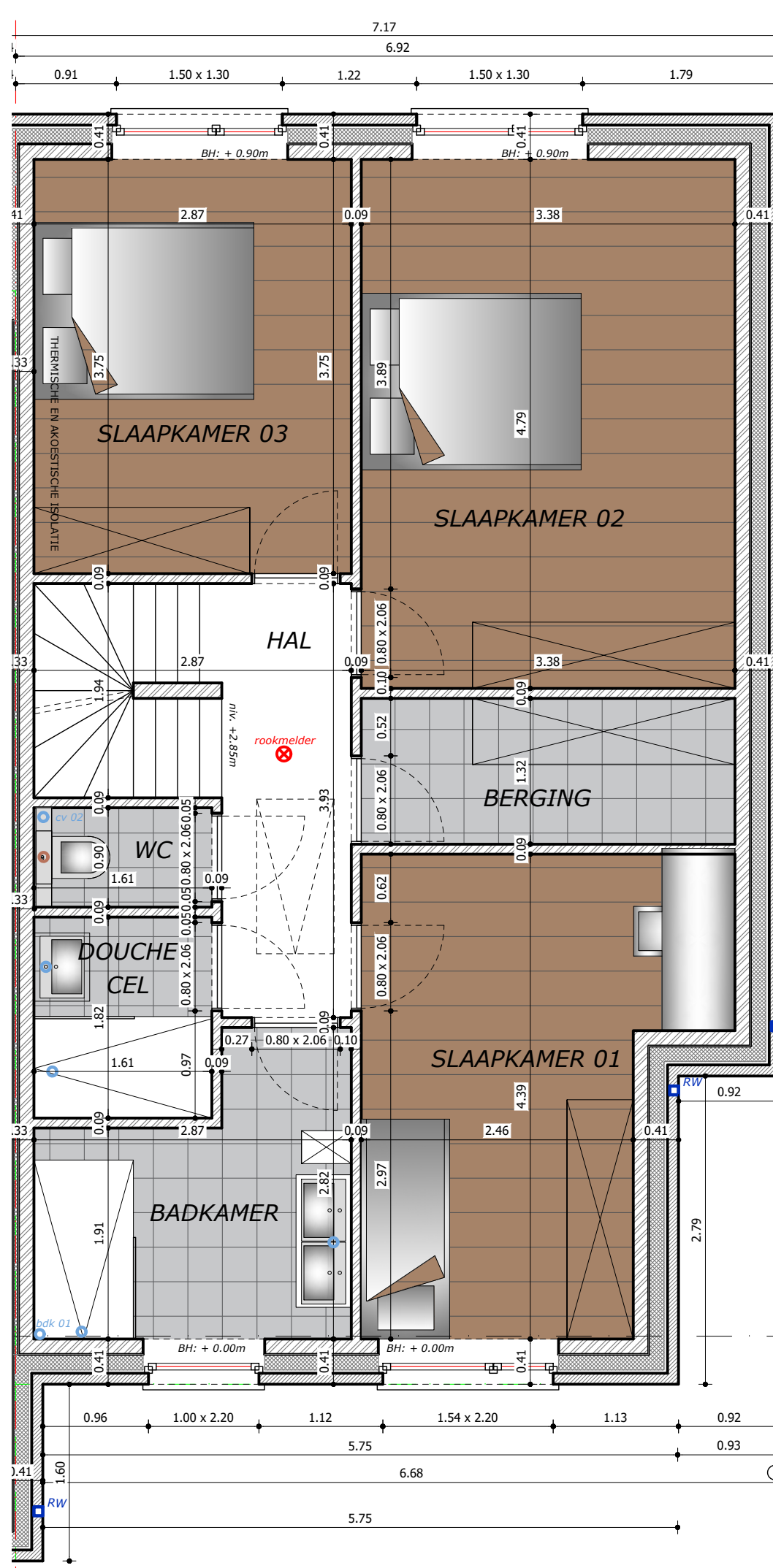
Verdieping 01
